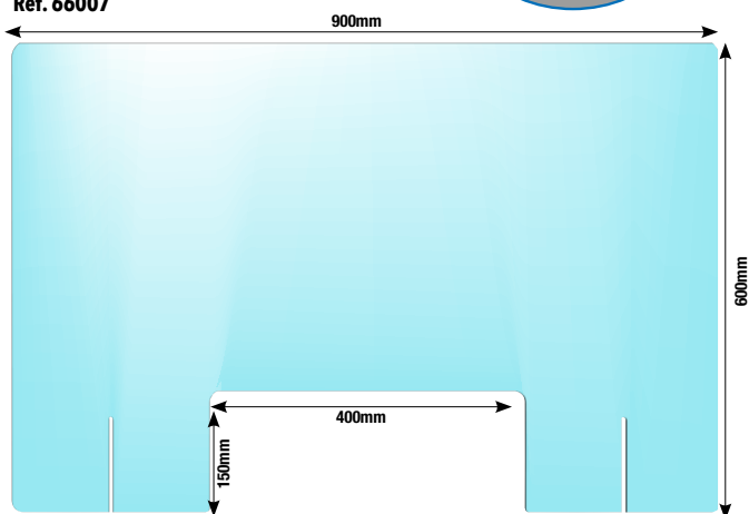
Réf. 66007
