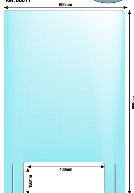
Réf. 66011
